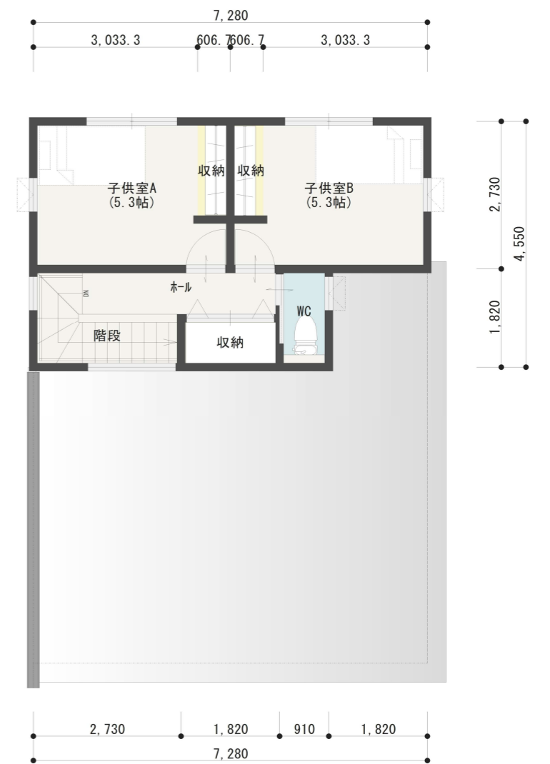
2F平面図
