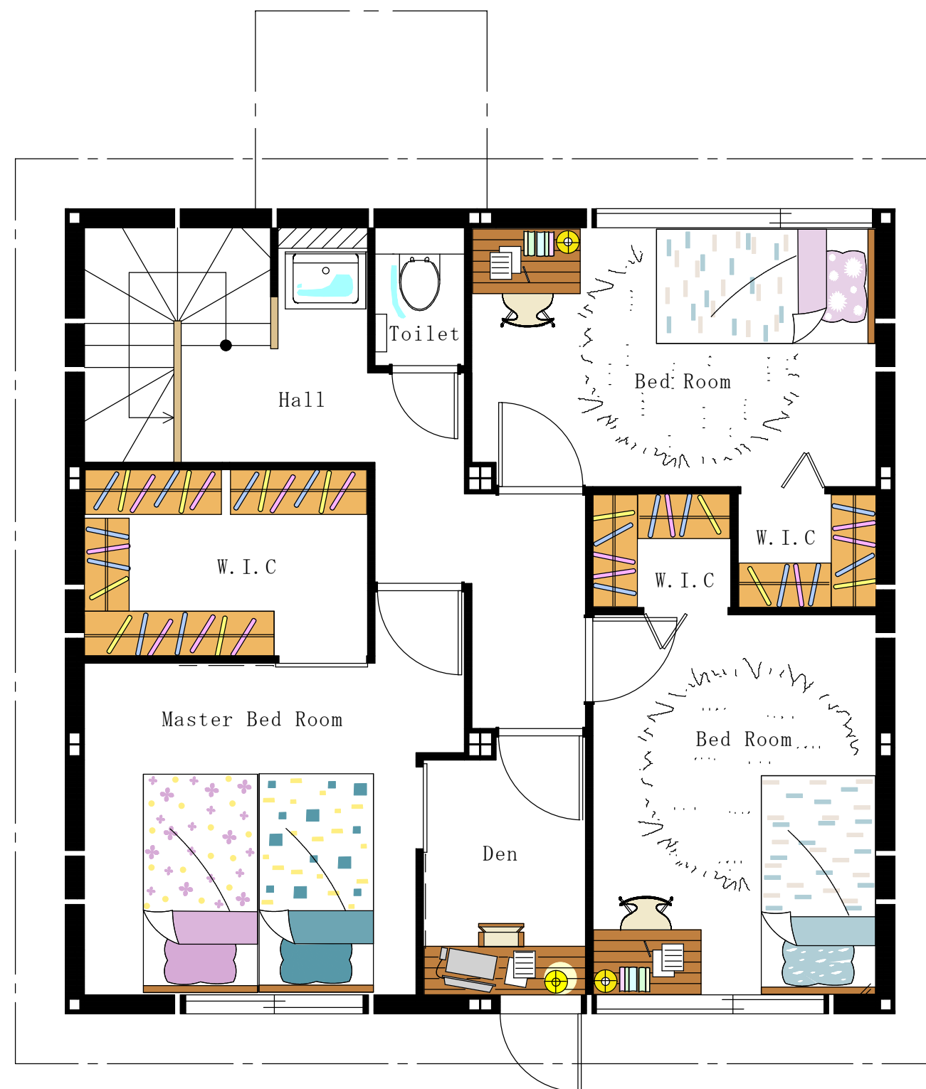
平面図 2階
