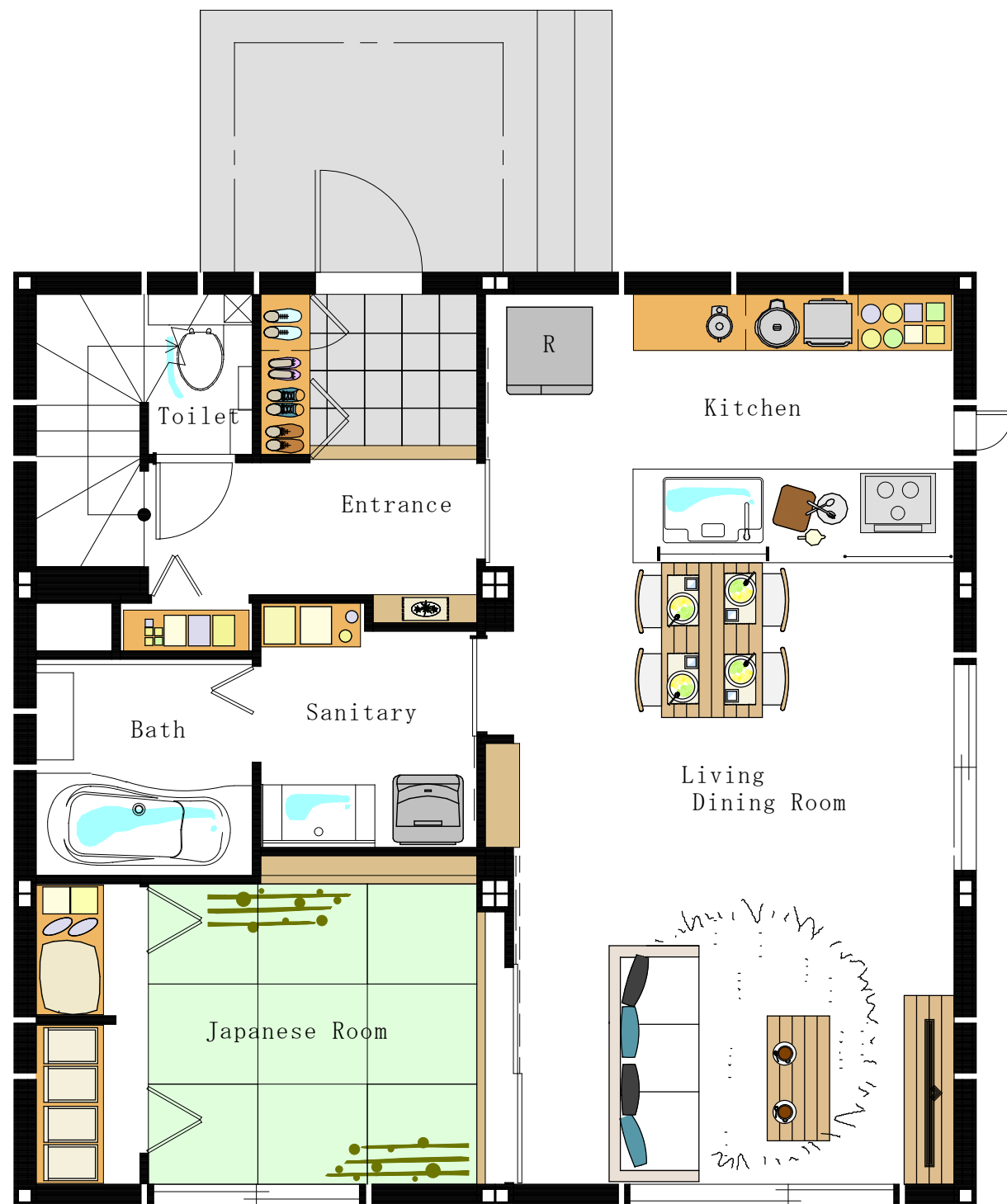
平面図 1階
